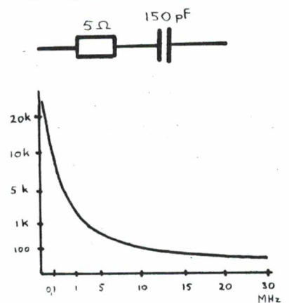
FIG. 11. De gemiddelde draadantenne gedraagt zich als een weerstand van 5 ohm in serie met een condensator van 150 pF. Dit geeft een zeer hoge impedantie op lagere frequenties
